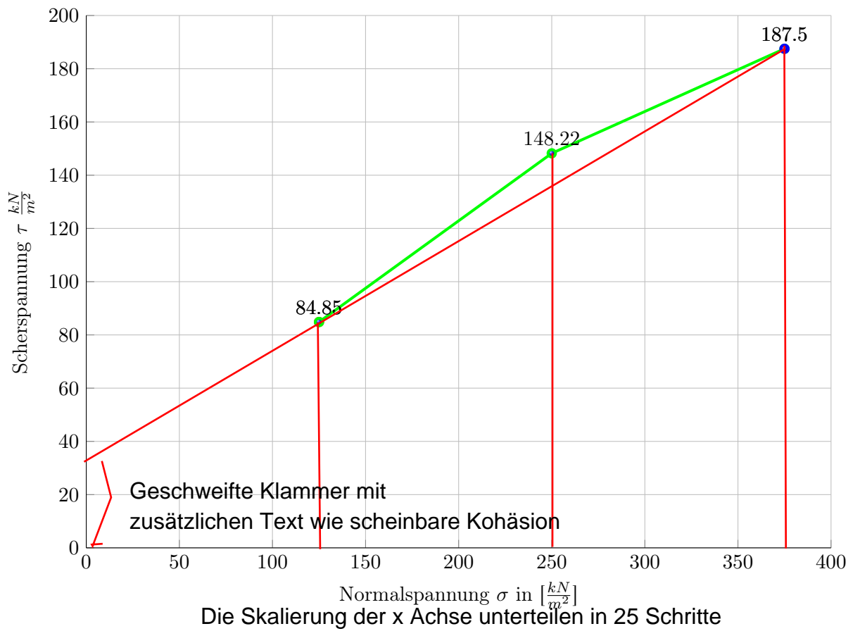
Figure 1: Normal-Scherspannungs - Diagramm
